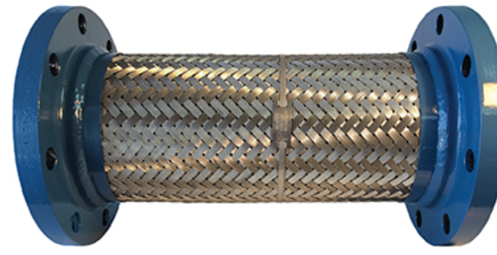
MFBA BRIDES #150 EN ACIER / CARBON STEEL 150# FLANGES
